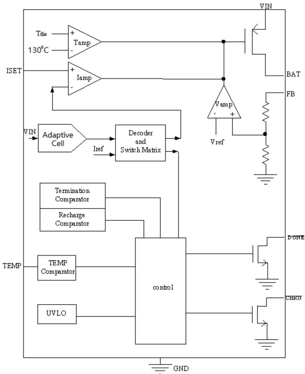
图 3 功能框图
